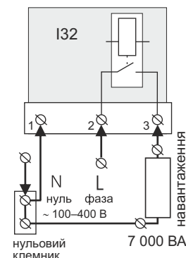
Схема 1. Спрощена внутрішня схема і схема підключення
