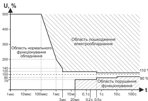
Рис. 1. Крива роботи електрообладнання ITIC (CBEMA), ( http://www.home.agilent.com/upload/cmc_upload/All/1.pdf?&cc=UA&lc=eng ).
